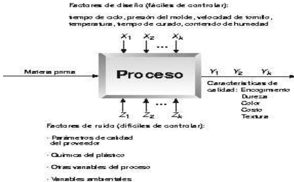
Figura 2. Aspectos de la planeación experimental en un ejemplo de producción de plástico.
